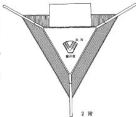
レストハウス平面図 1/200
