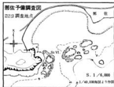
保護詳細計画図 3
