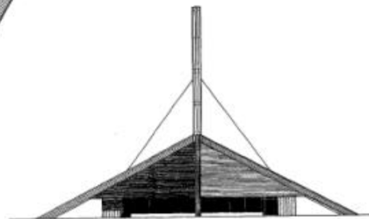
レストハウス西立面図 1/200
